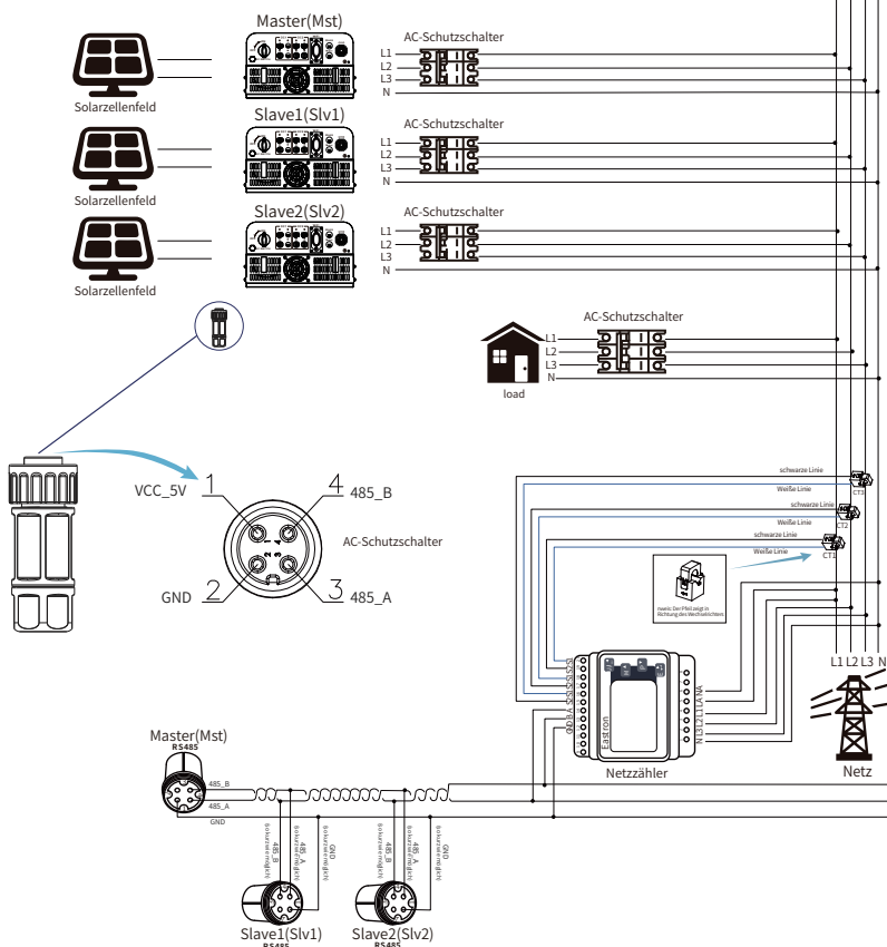
Abb. 7.23 Anschlussplan (Dreiphasenstrom)
