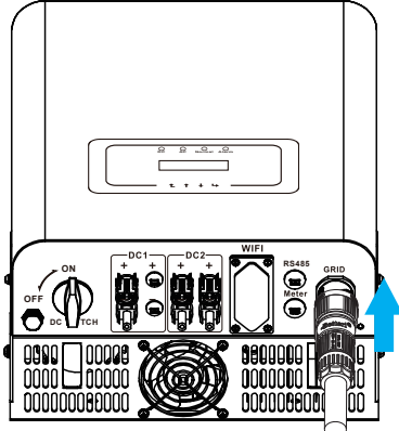
Abb. 5.10 AC-Eingangsanschluss
