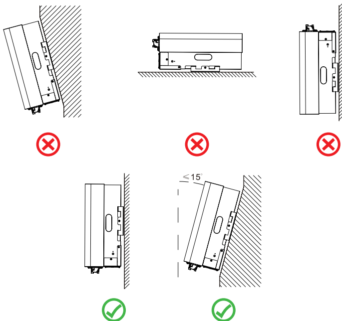
Abb. 4.2 Einbauwinkel
