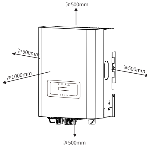
Abb. 4.3 Einbaulücke
