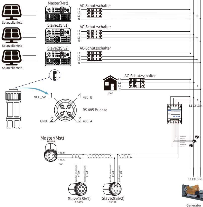
Abb. 7.33 CHINT Anschlussplan (Die Durchleitungstabelle)
